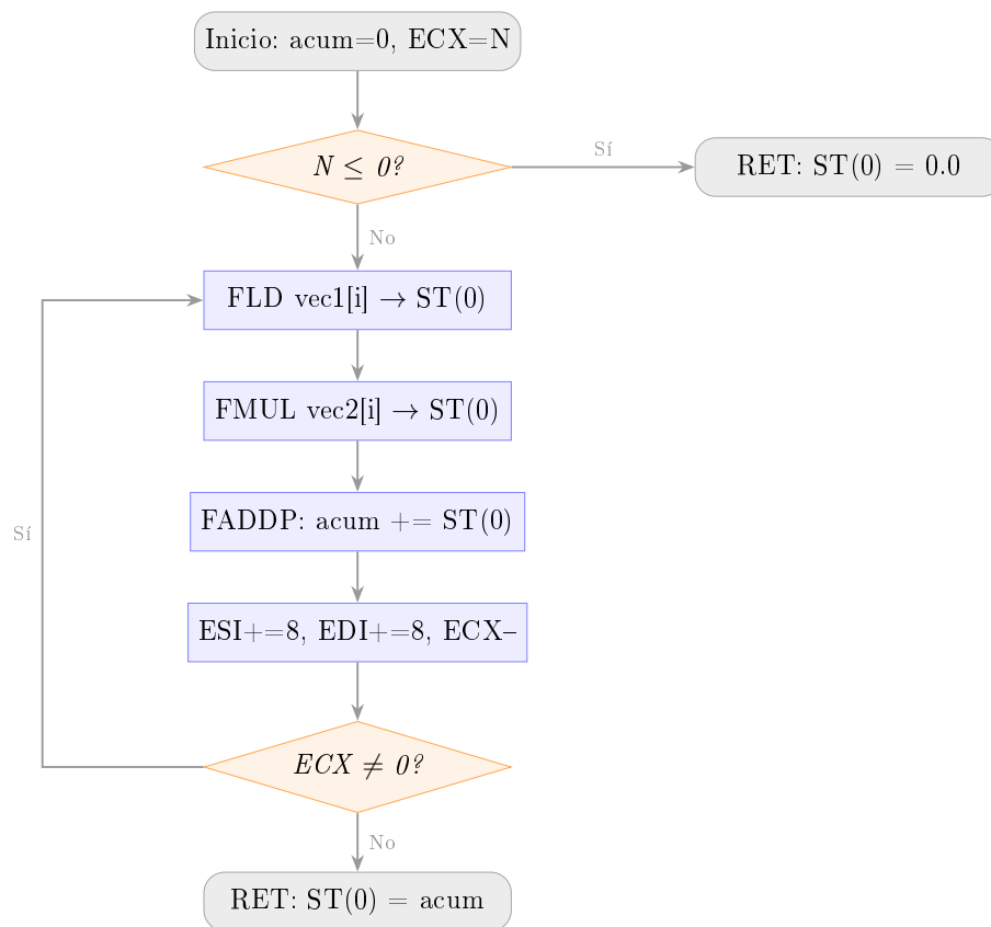
Figura 1: Diagrama de flujo del algoritmo de producto punto
