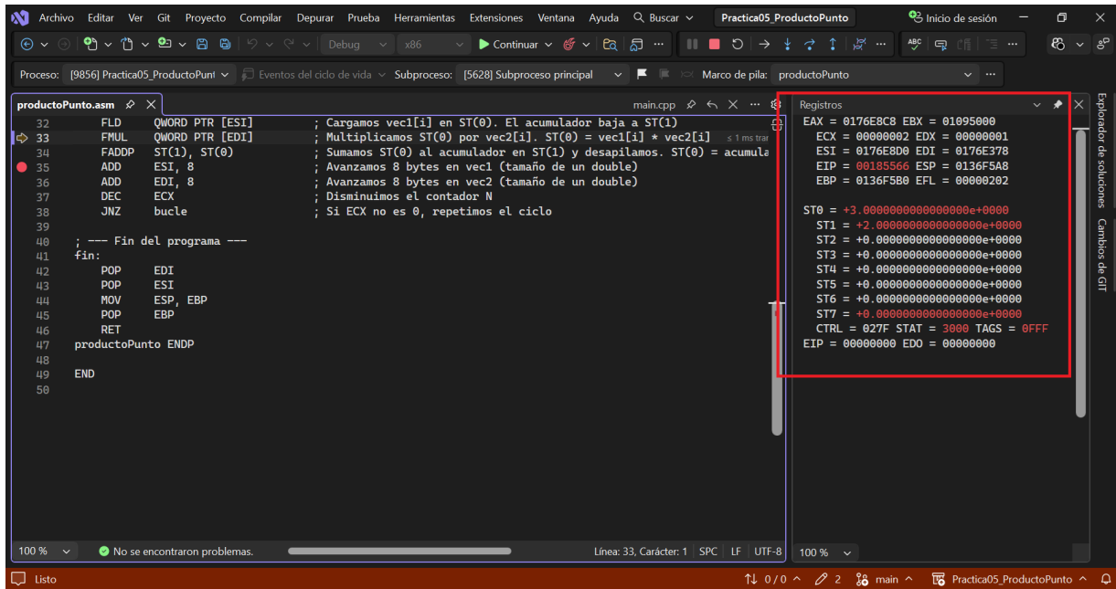
Figura 2: Ventana Registers de Visual Studio: registros FPU ST(0)–ST(7) y ECX durante el bucle de acumulación.
